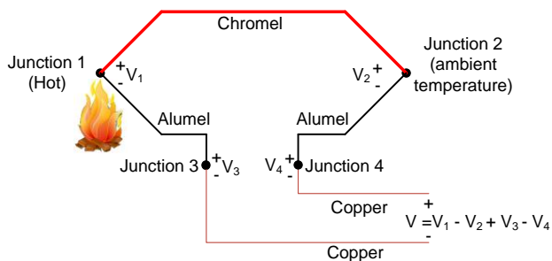
图 5. 测量热电势
