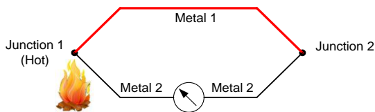
图 1(b). 热电偶 — 塞贝克(Seebeck)效应
